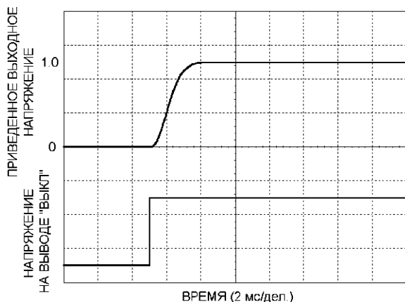
Рис. 15. Типовой процесс включения по входу "ВЫКЛ"
