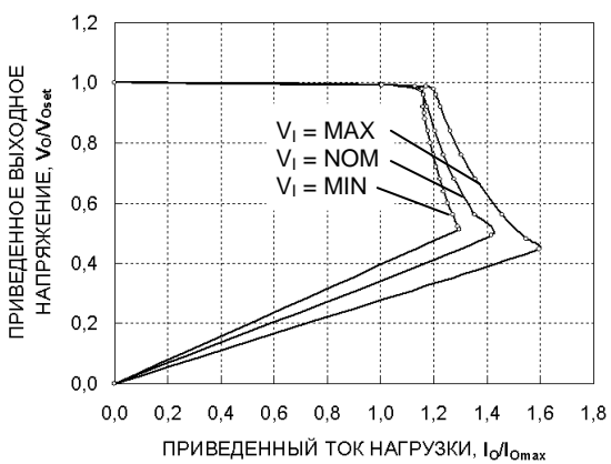
Рис. 3. Зависимость выходного напряжения от тока нагрузки при T_c=25^\circ C
