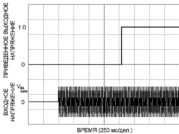
Рис. 14. Типовой процесс включения при подаче питания
