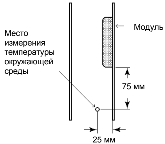
Рис. 31. Установка для измерения перегрева корпуса
