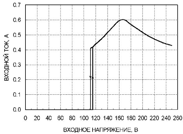
Рис. 1. Зависимость входного тока от входного напряжения для модулей МПС60 при I_o = I_{o,max} и T_c=25^\circ C
