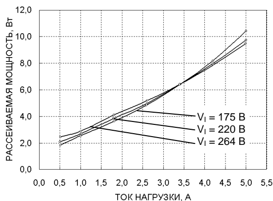
Рис. 26. Типовая зависимость рассеиваемой мощности от тока нагрузки для модуля МПС60В при T_c=25^\circ\text{C}
