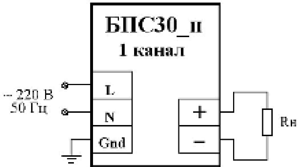
Рисунок Д.1 – Типовая схема включения блоков
