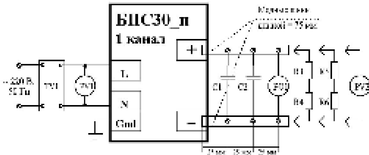
Рисунок Г.1 – Схема проверки амплитуды пульсации выходного напряжения
