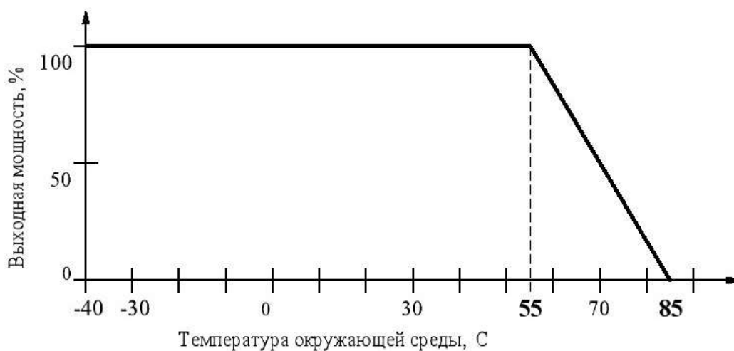
Рисунок Е.2 – Зависимость выходной мощности от температуры окружающей среды в условиях естественной конвекции (для К.П.Д. = 85 %)
