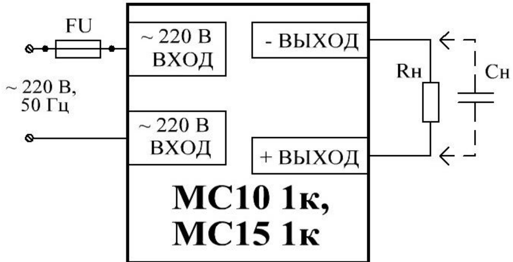
Рисунок Д.2 – Типовая схема включения модулей серий MC10, MC15
