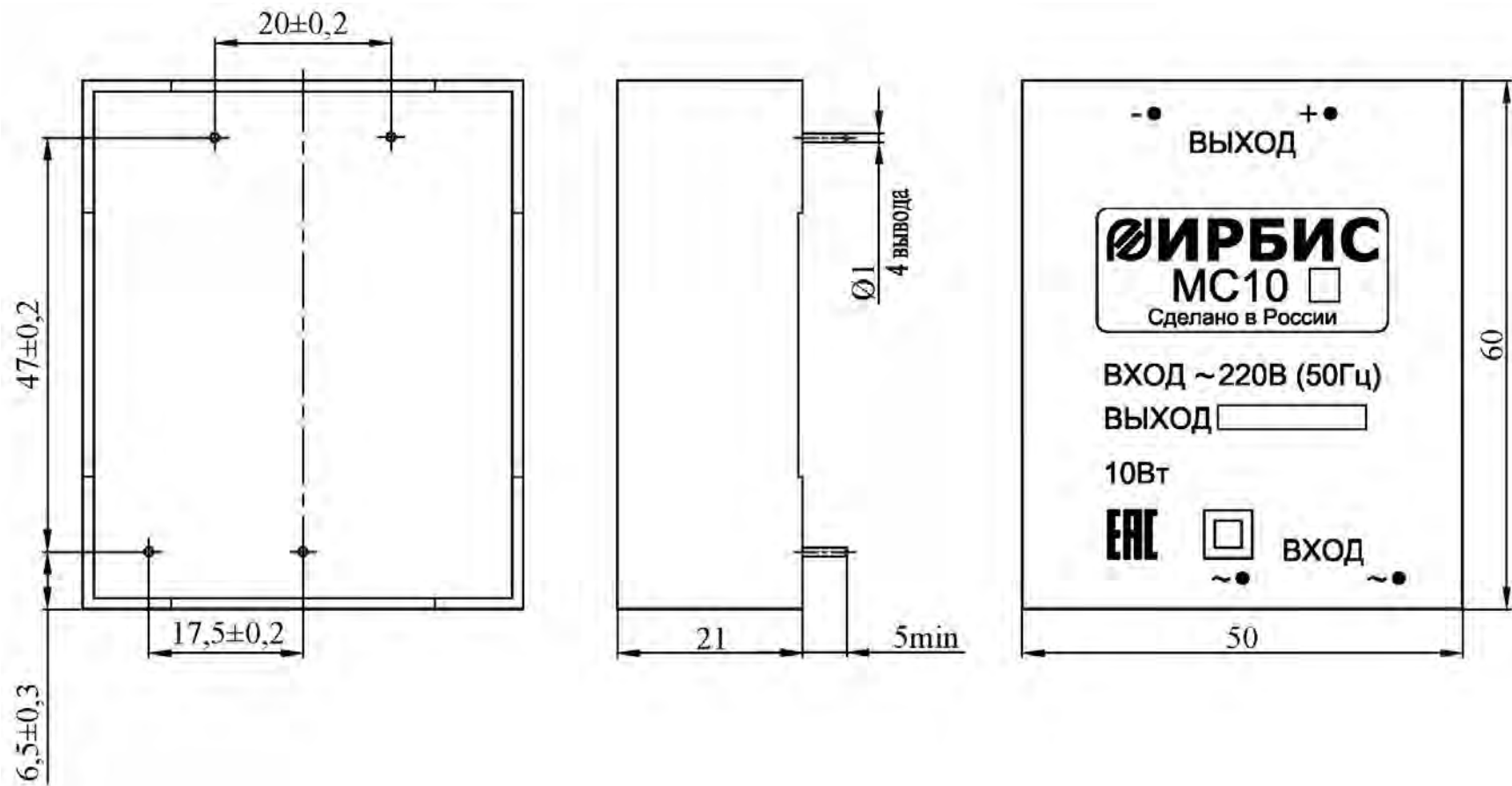
Рисунок В.2 – Габаритный чертеж модулей серии MC10_
