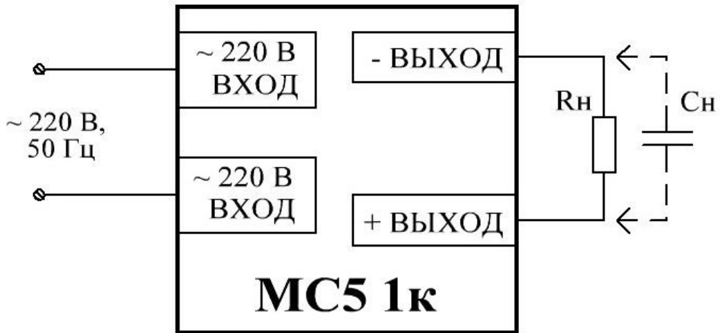
Рисунок Д.1 – Типовая схема включения модулей серии MC5
