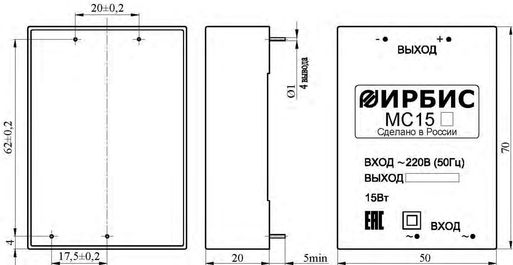
Рисунок В.3 – Габаритный чертеж модулей серии MC15_
