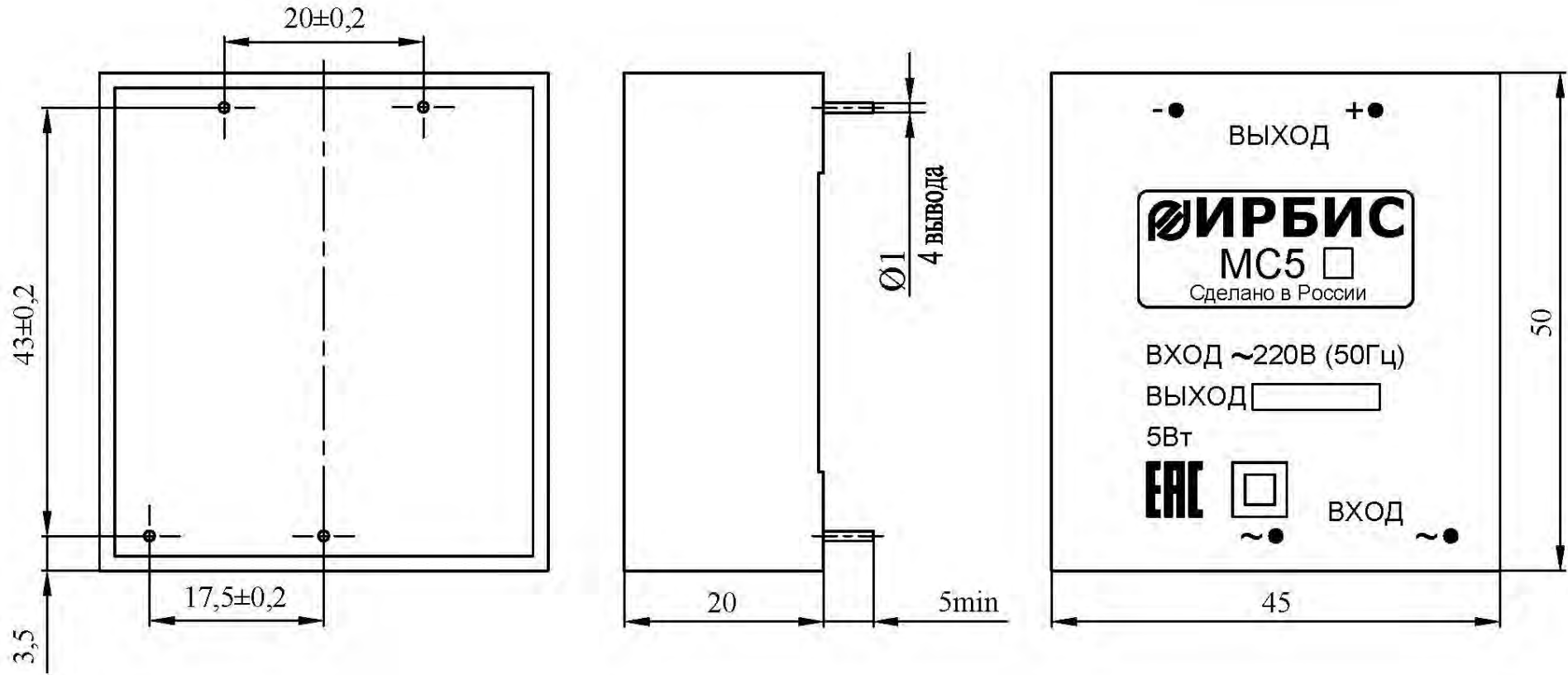
Рисунок В.1 – Габаритный чертеж модулей серии MC5_
