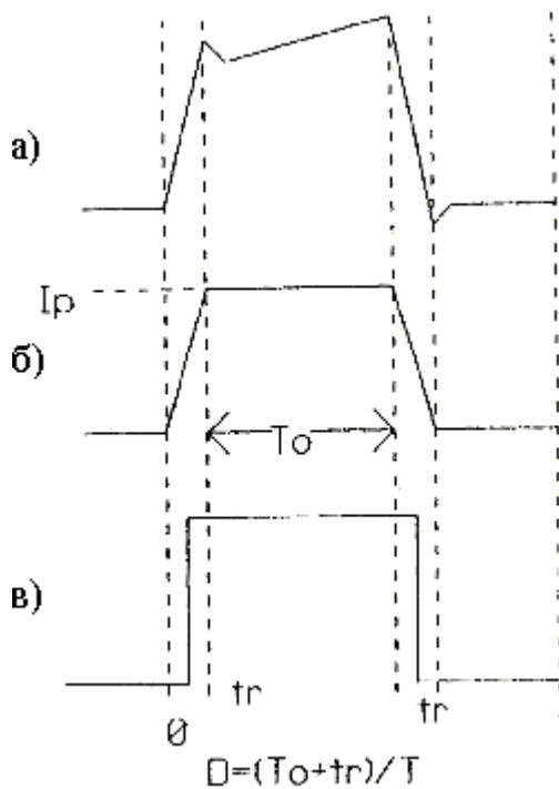
Рис. 1. Типовая форма тока в трансформаторах одноктных преобразователей с эквивалентными аппроксимациями.
