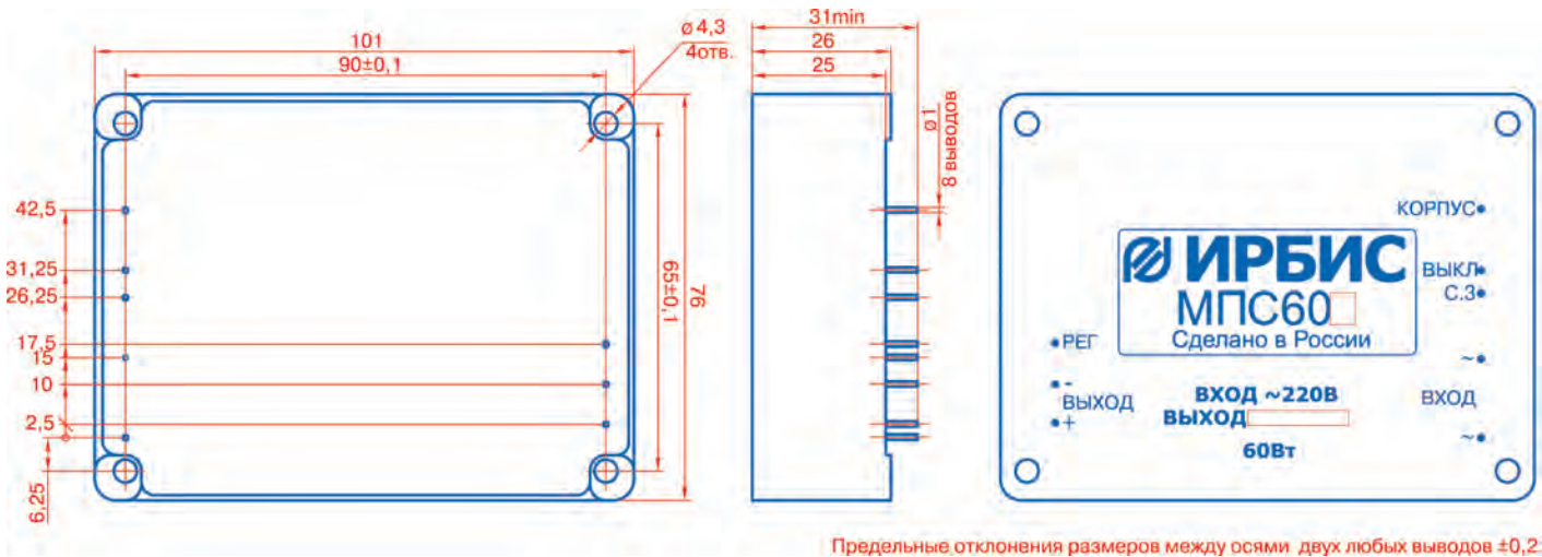
Предельные отклонения размеров между осями двух любых выводов ±0,2
