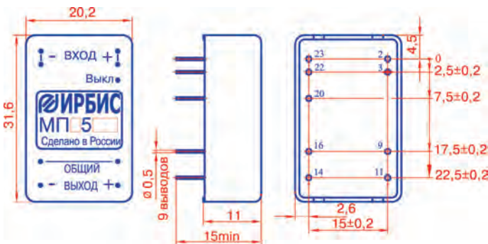
Маркировка выводов показана условно
