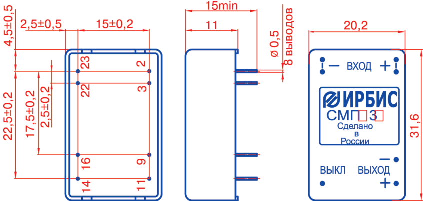
Номера выводов показаны условно Вывод “9” – не задействован
