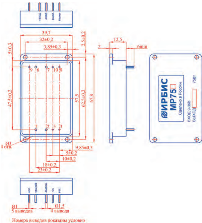
Номера выводов показаны условно
