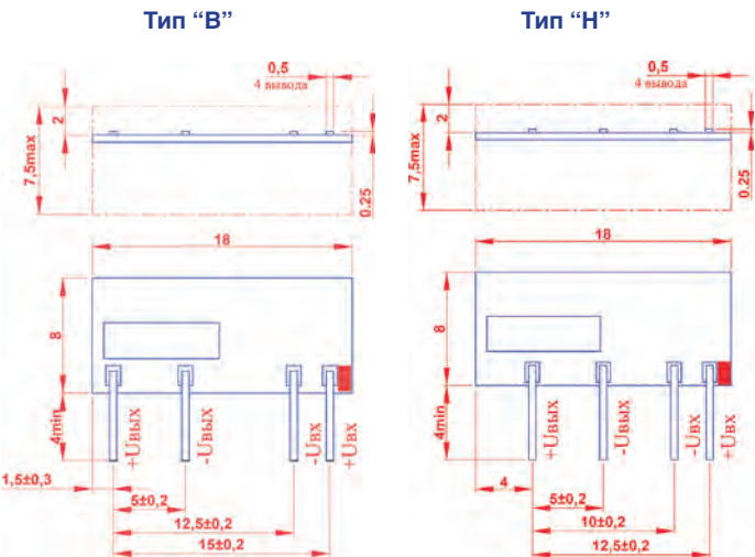
Маркировка выводов показана условно
