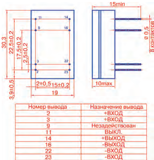
Номера выводов показаны условно
