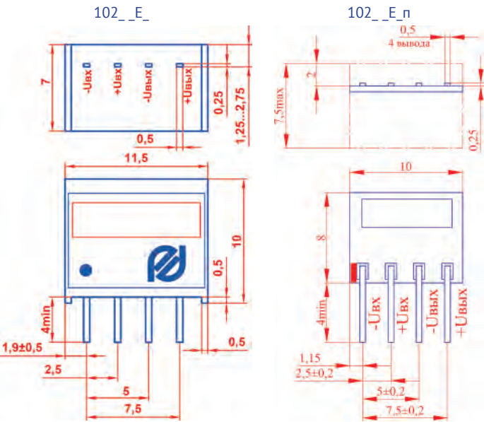
Маркировка выводов показана условно
