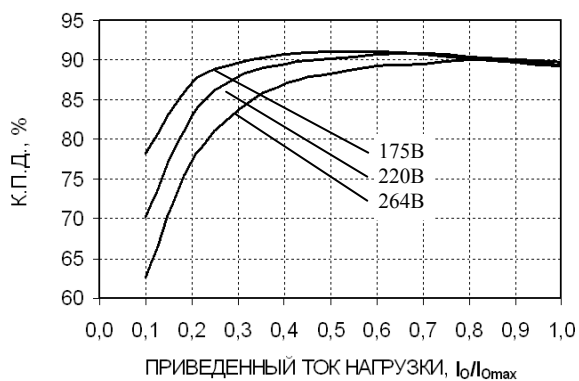
Рис. 7. Типовая зависимость К.П.Д. от тока нагрузки для модуля БПС200Б при T_c=25^\circ\text{C}
