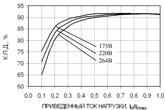
Рис. 8. Типовая зависимость К.П.Д. от тока нагрузки для модуля БПС200Е при T_c=25^\circ\text{C}
