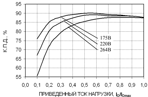
Рис. 6. Типовая зависимость К.П.Д. от тока нагрузки для модуля БПС 200А при T_c=25^\circ\text{C}
