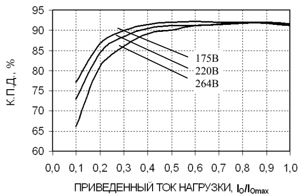
Рис. 9. Типовая зависимость К.П.Д. от тока нагрузки для модуля БПС200Н при T_c=25^\circ\text{C}
