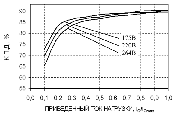
Рис. 10. Типовая зависимость К.П.Д. от тока нагрузки для модуля БПС200У при T_c=25^\circ\text{C}
