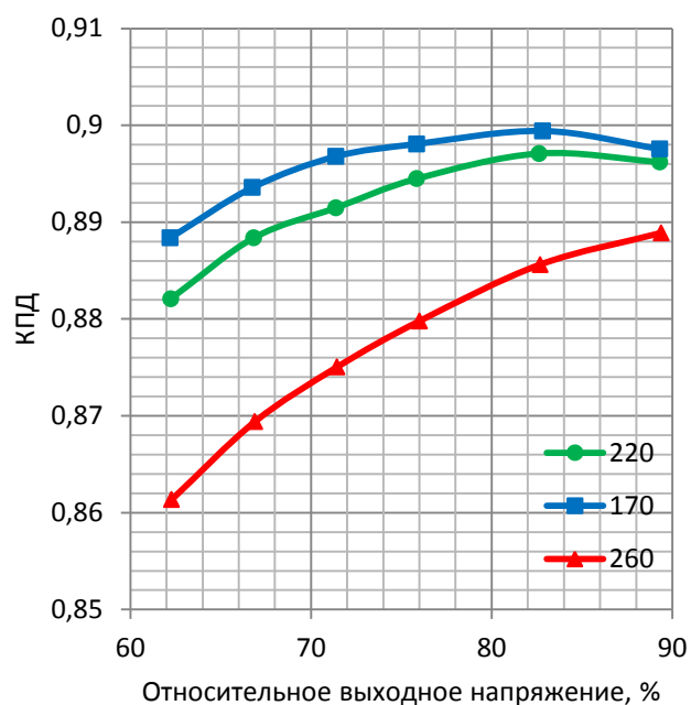
Зависимость коэффициента полезного действия от выходного напряжения
