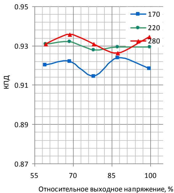
Зависимость коэффициента полезного действия от выходного напряжения
