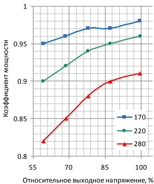
Зависимость коэффициента мощности от выходного напряжения
